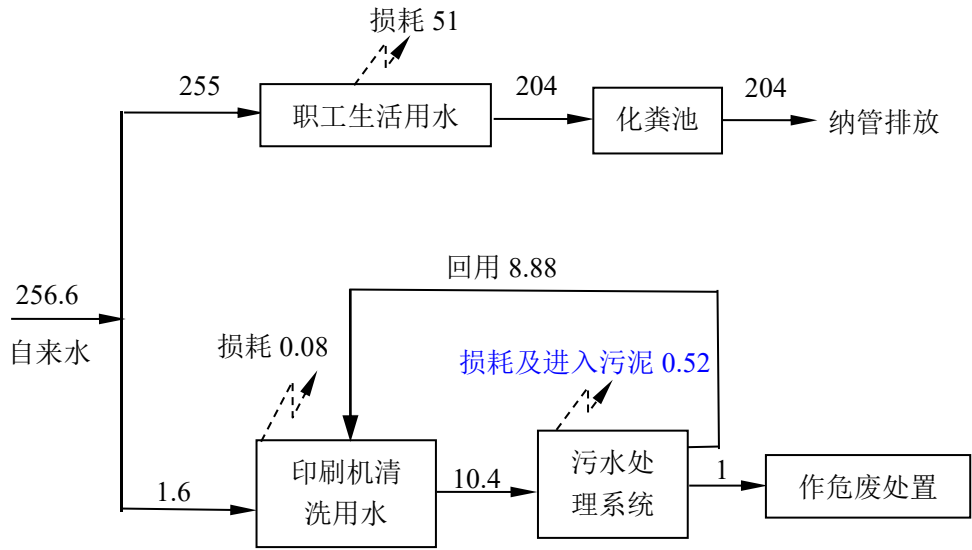
图 2-7 本项目水平衡图 t/a
