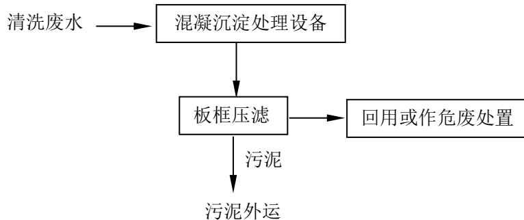
图 4-1 清洗废水处理工艺流程图
