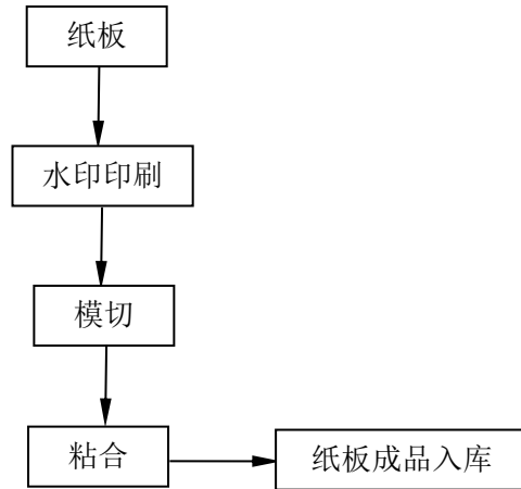
图 2-11 纸板工艺流程及产污环节图
