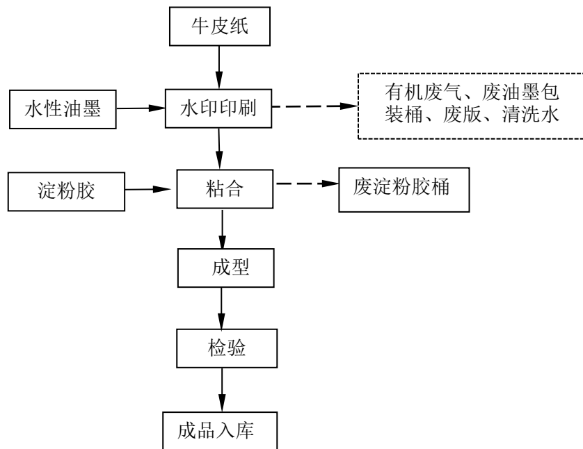
图 2-9 牛皮纸袋工艺流程及产污环节图
