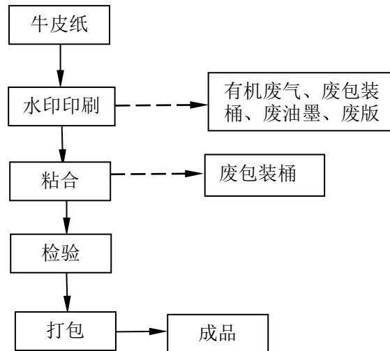
图 2-12 牛皮纸袋工艺流程及产污环节图
