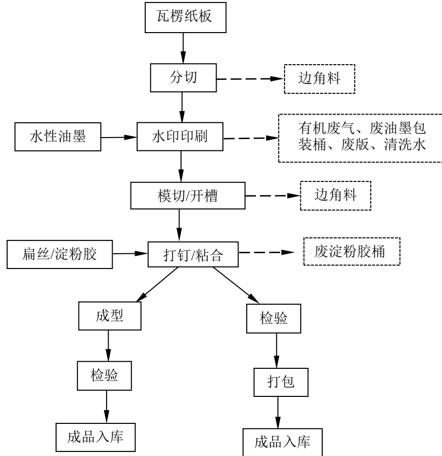
图 2-8 纸板（纸箱）工艺流程及产污环节示意图
