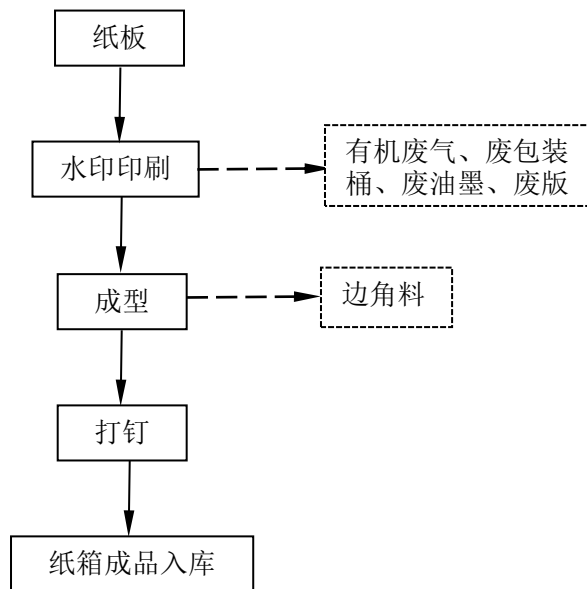
图 2-10 纸箱工艺流程及产污环节图
