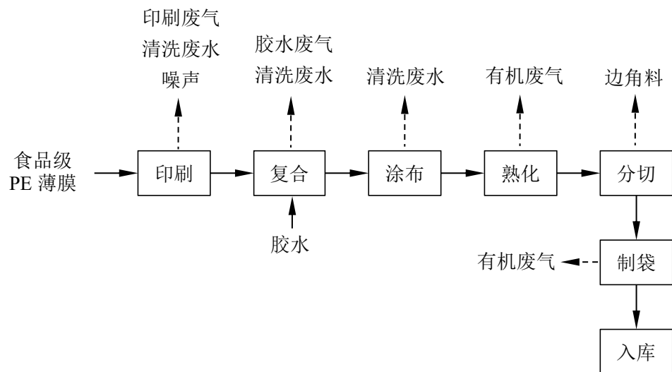
图 2-7 塑料类包装材料生产工艺流程及产污环节示意图
