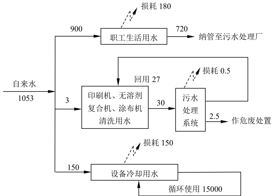
图 2-4 本项目水平衡图 t/a
