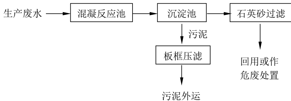
图 4-1 污水处理系统废水处理工艺流程图
