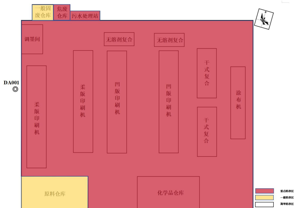
图 4-3 企业厂区分区防渗图
